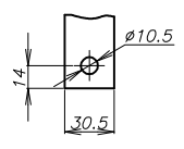
접속도체 가공도
