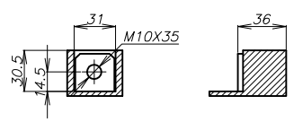
단자부 상세도
