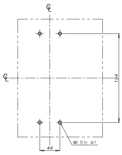
패널설치치수
